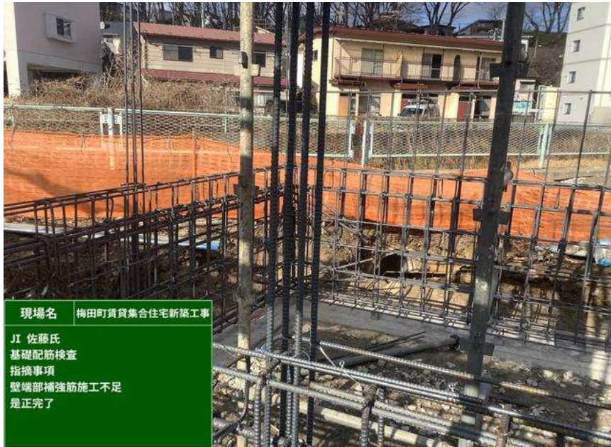
現場名 梅田町賃貸集合住宅新築工事 JI 佐藤氏 基礎配筋検査 指摘事項 壁端部補強筋施工不足 是正完了
